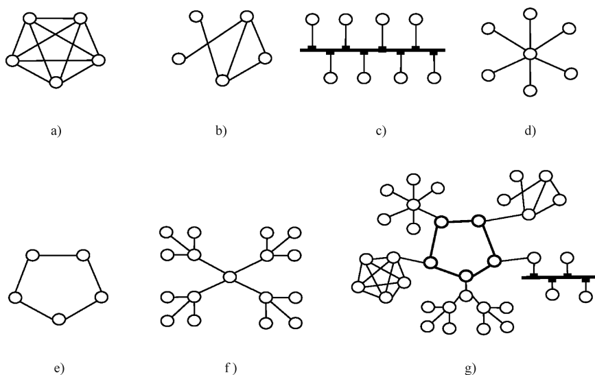
图 2.1 网络拓扑
