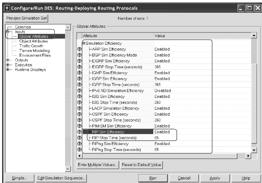
图 11.9 指定 RIP 仿真效率模式
