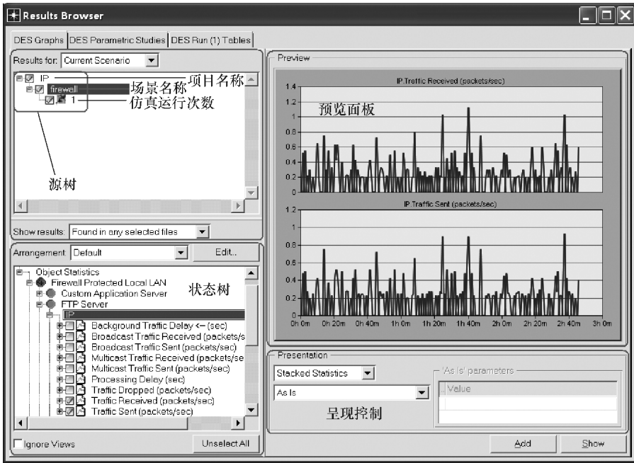
图 4.11 Results Browser 窗口的 DES Graphs 选项卡
