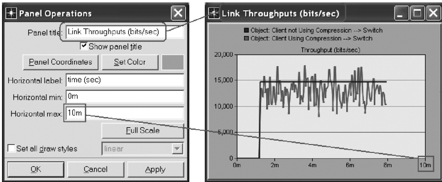
图 4.22 一个 Panel Operations 窗口及其图形
