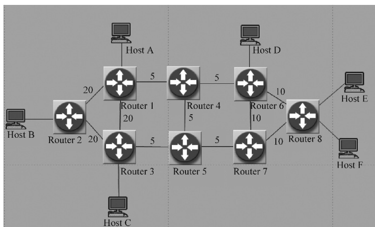
图 L12.1 OSPF 研究的网络拓扑
