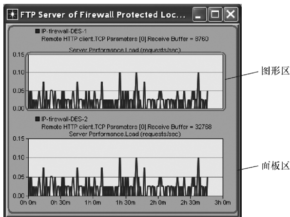
图 4.14 在图 4.12 中选中统计量的分析平板
