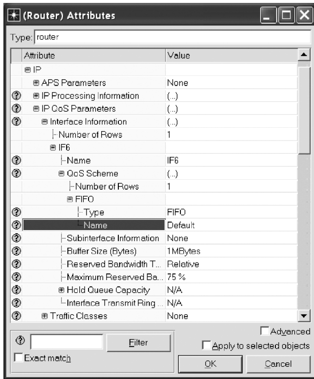
图 L10.2 支持 FIFO QoS 方案的 Router 配置例子
