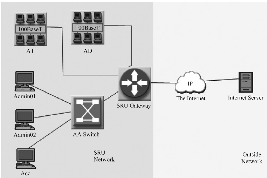
图 L9.1 这项作业的网络拓扑
