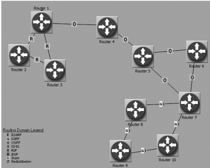
图 11.3 路由协议部署范例
