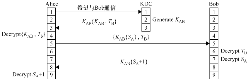
图 L5.1 Secure AB talk 认证协议
