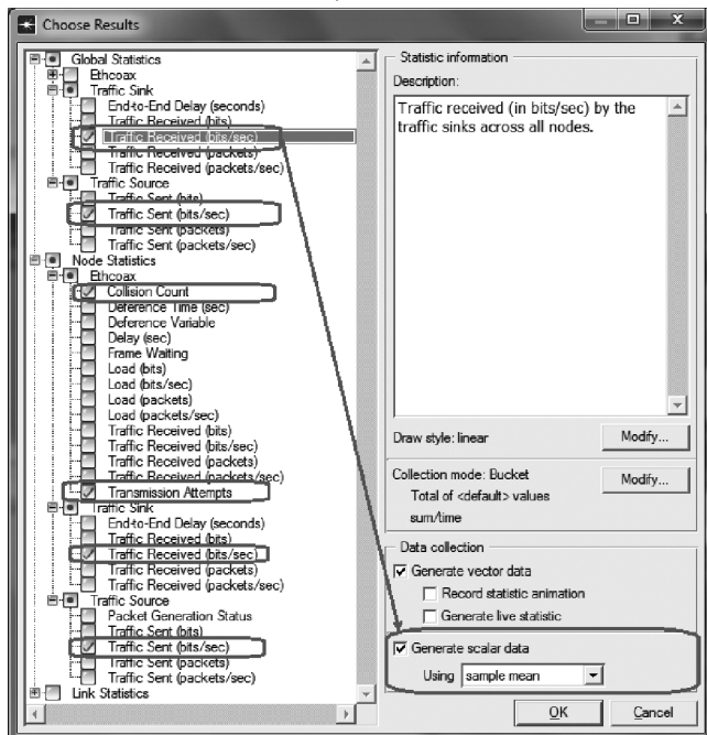
图 L13.2 配置仿真收集标量统计量
