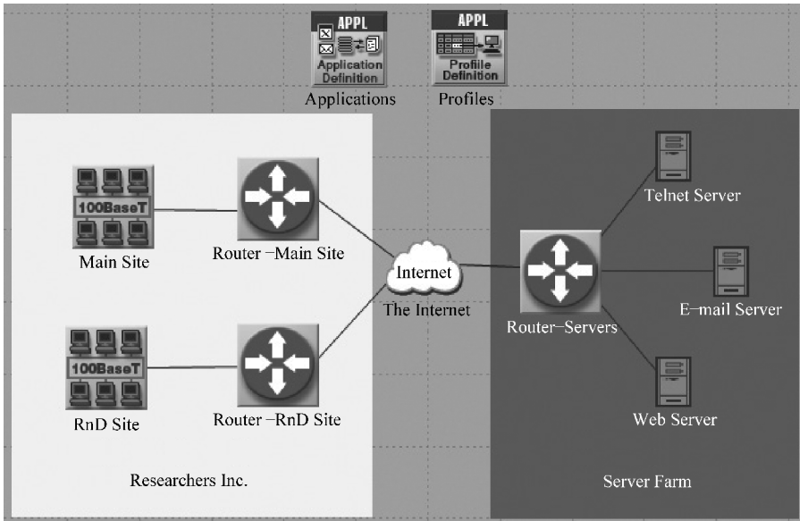
图 L3.1 这项作业的网络拓扑
