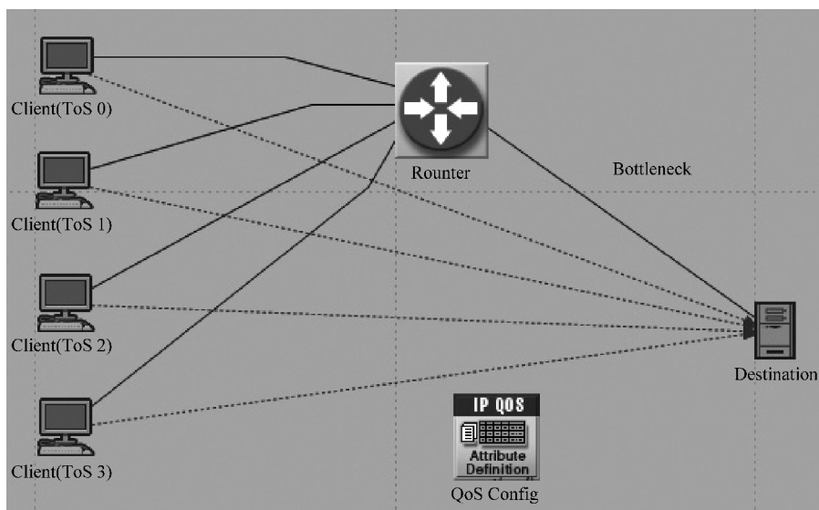
图 L10.1 网络拓扑
