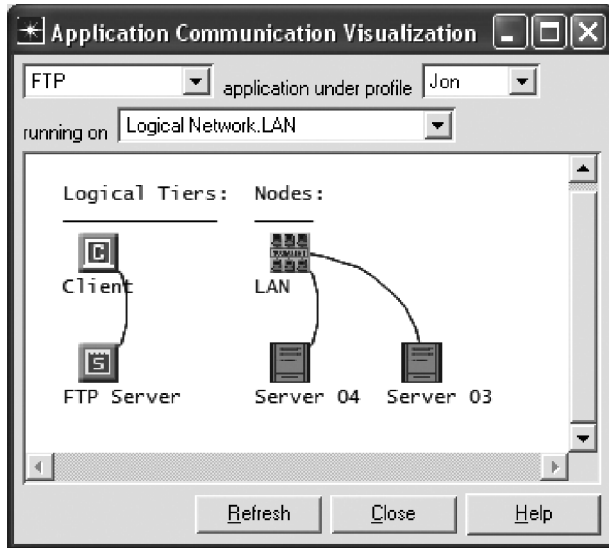
图 7.14 Application Communication Visualization (应用通信可视化) 窗口
