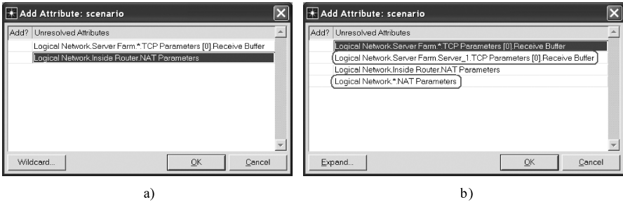
图 3.12 Add Attribute 窗口
