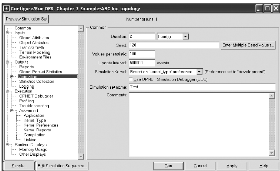
图 4.6 Configure/Run DES 窗口的详细视图
