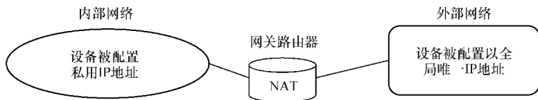
图 10.1 带有一台支持 NAT 的路由器的范例网络拓扑
