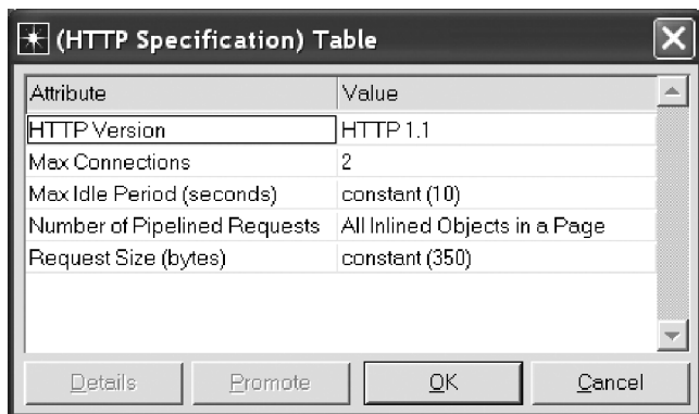
图 5.10 HTTP 规格复合属性
