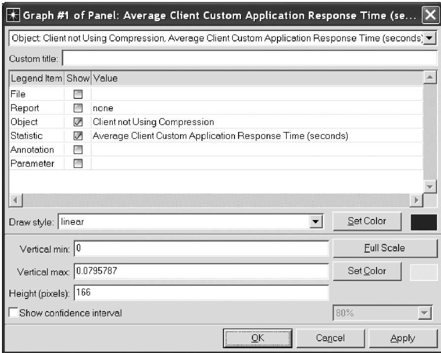
图 4.24 Edit Graph Properties 窗口
