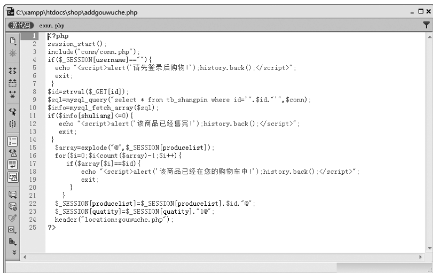
图 9-41 addgouwuche.php 页面的设计
