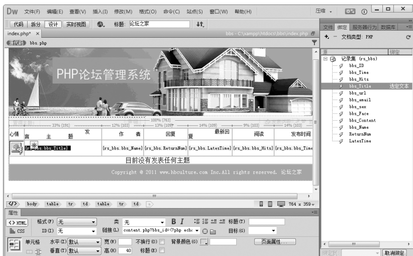
图 8-24 字段插入至 index.php
