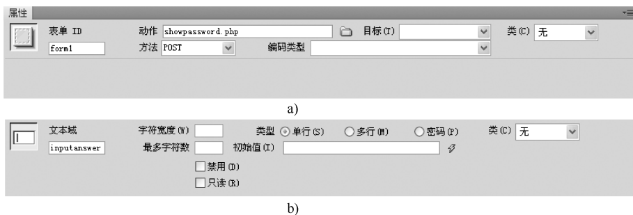
图 4-74 设置表单提交的属性
