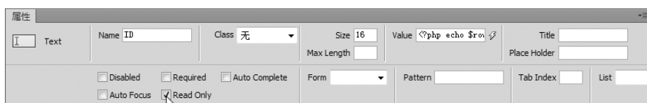
图 3-80 设置为“只读”属性
