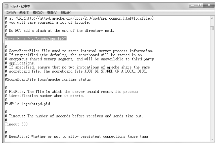
图 1-33 设置网站文件位置
