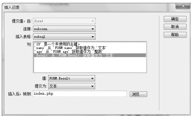
图 3-67 设置“插入记录”对话框
