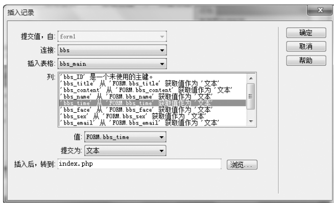
图 8-59 设定“插入记录”
