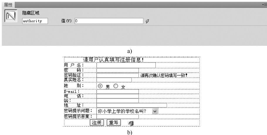
图 4-47 register.php 页面静态设计
