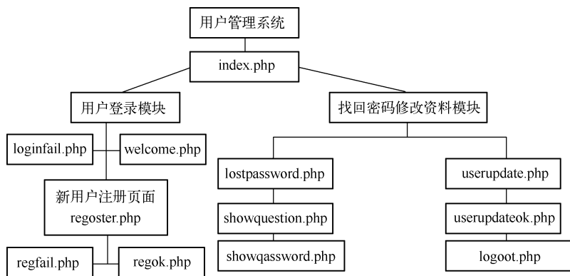
图 4-1 系统结构图
