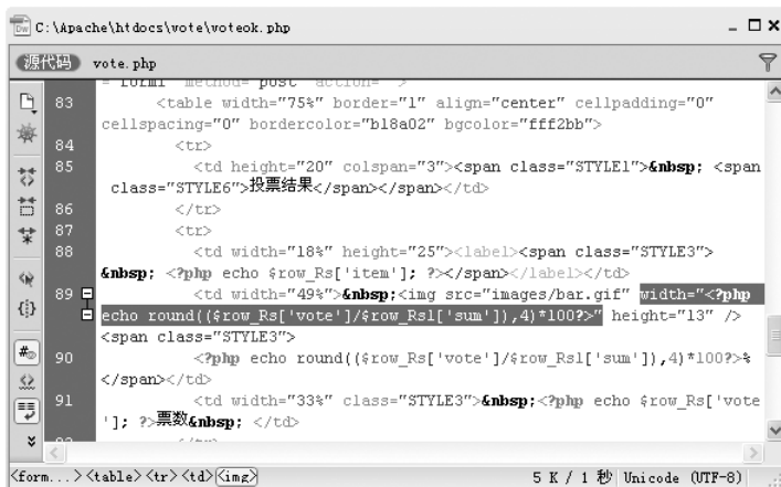
图 7-35 设置图像的缩放
