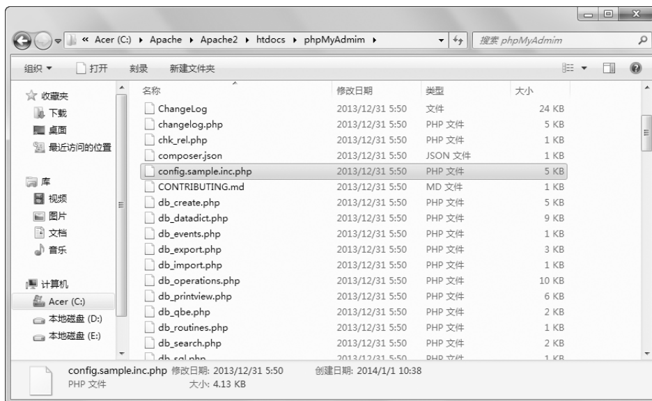
图 1-71 创建 config.inc.php 文件
