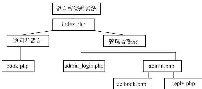
图 6-1 系统结构图
