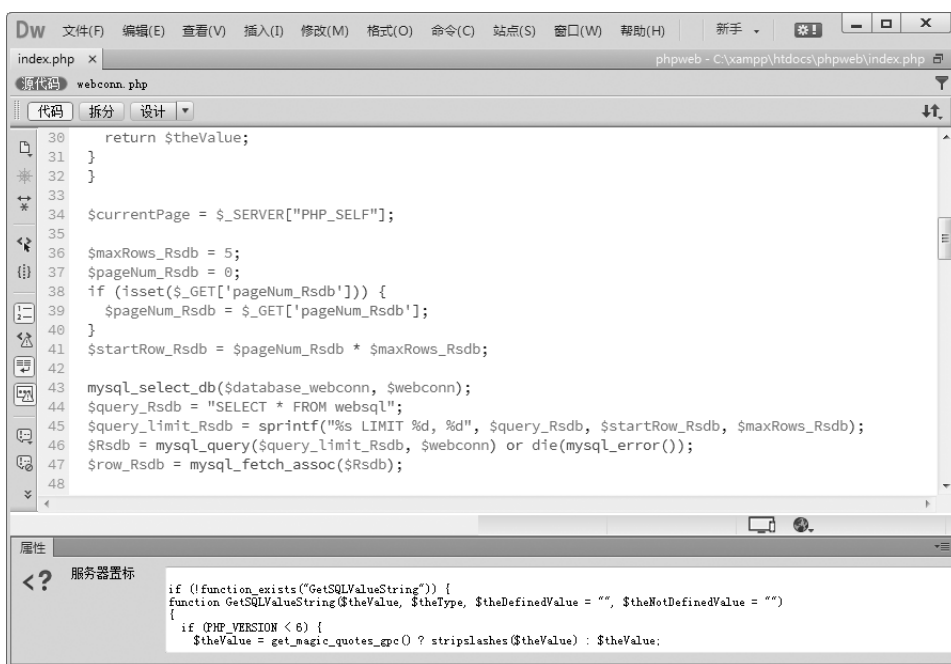
图 3-72 代码窗口
