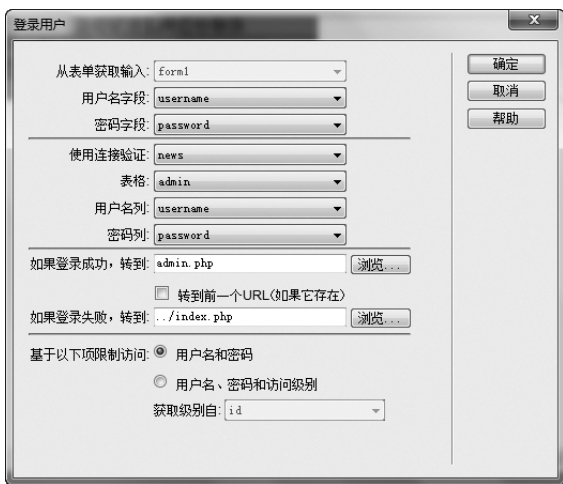
图 5-63 设置“登录用户”对话框
