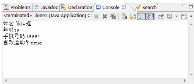
图 9-1 类的继承
