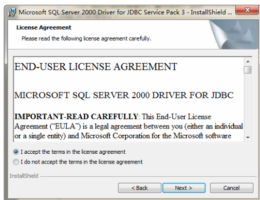
图 19-18 遵守协议
