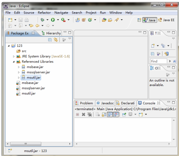
图 19-26 加载驱动
