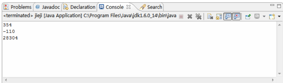
图 9-19 接口的继承
