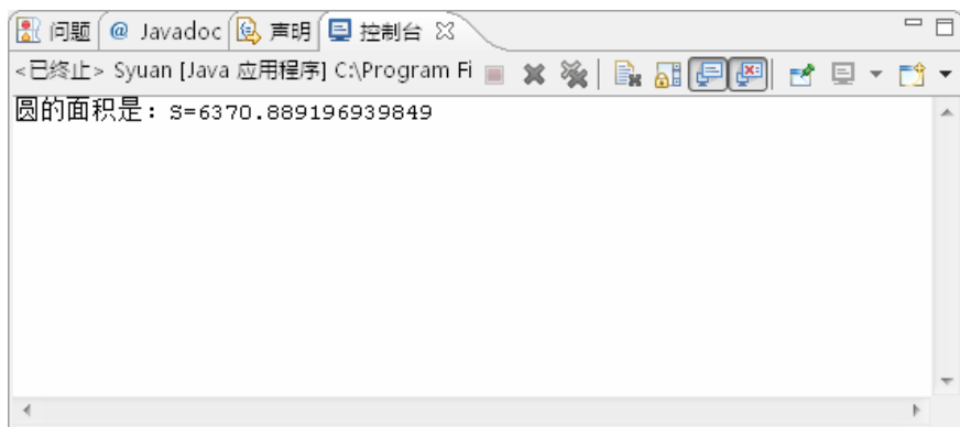
图 3-9 浮点型数据
