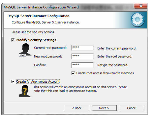
图 16-20 设置密码
