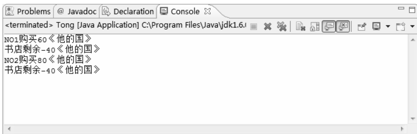
图 12-14 线程同步
