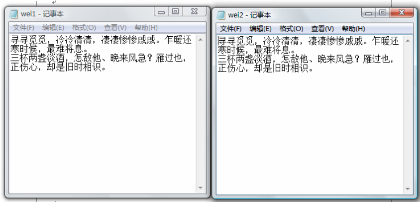
图 11-10 执行结果
