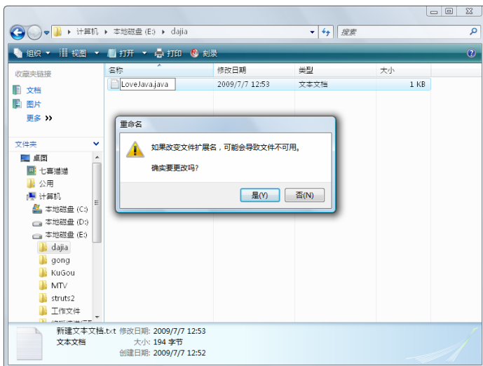
图 1-20 重命名
