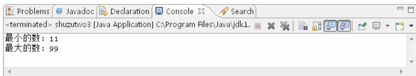
图 7-9 执行结果
