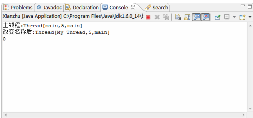
图 12-2 创建主线程
