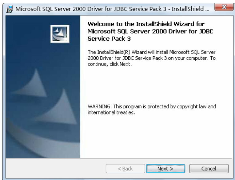
图 17-9 第一个向导
