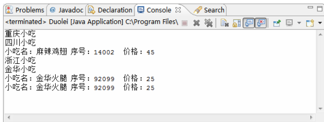
图 9-7 多重复继承
