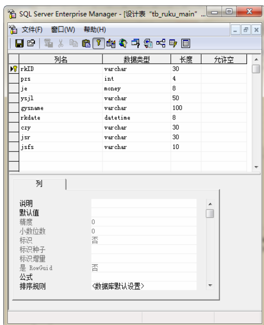
图 19-8 入库主表
