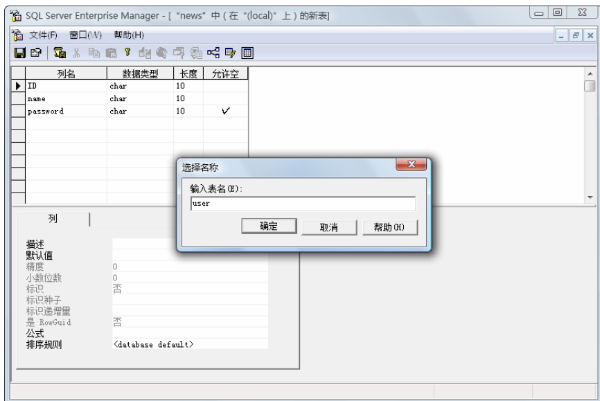
图 16-37 输入表名
