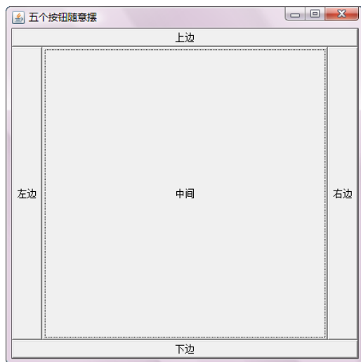
图 14-8 BorderLayout 布局
