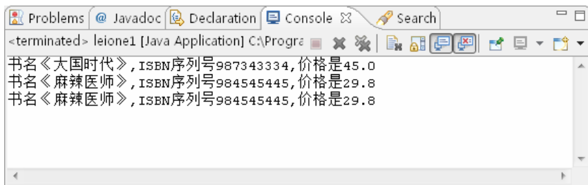
图 8-4 执行结果
