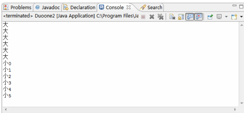
图 12-5 创建线程
