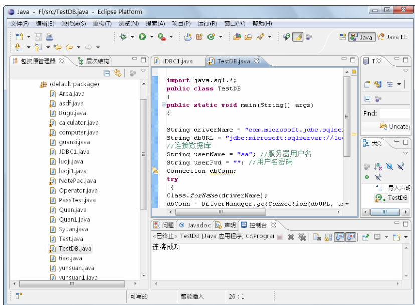
图 17-16 连接成功
