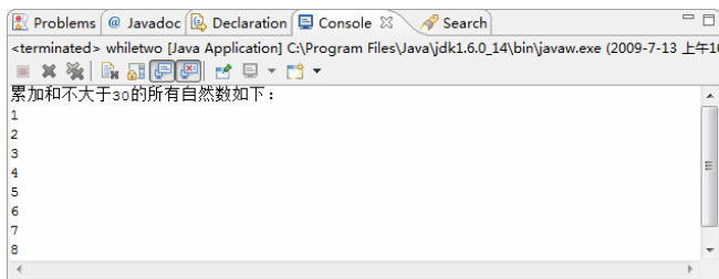
图 6-11 累加的和
