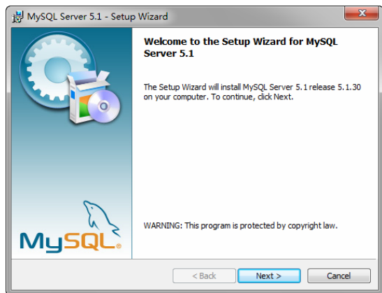
图 16-8 安装向导
