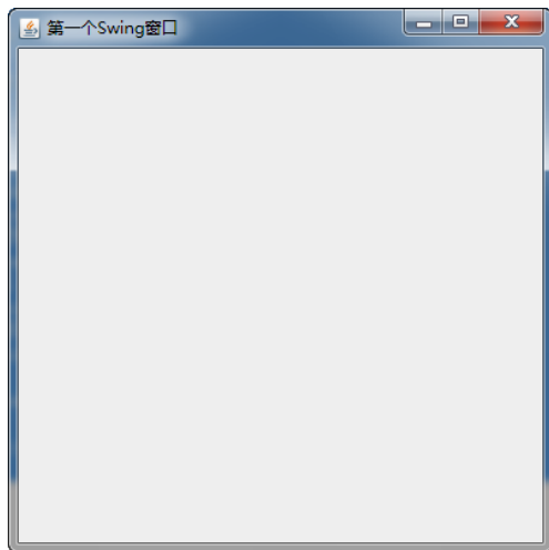
图 15-2 Swing 窗口
