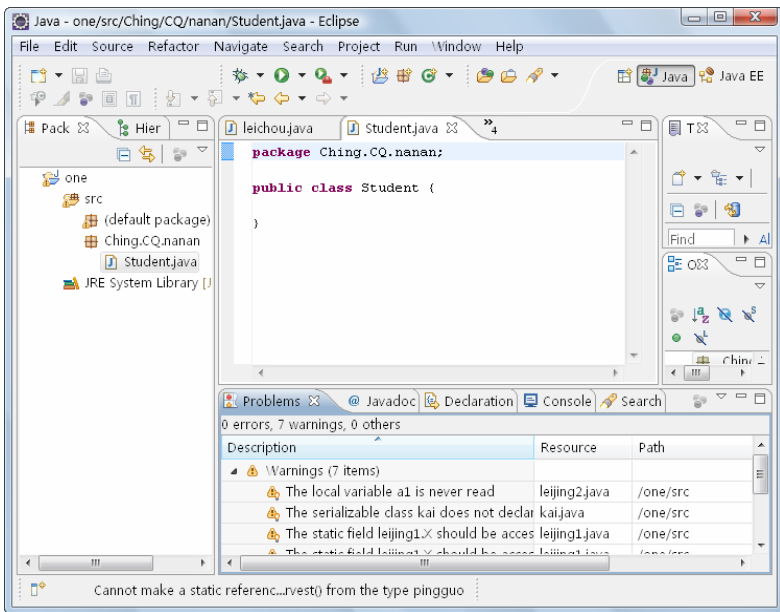
图 8-22 新建的包
