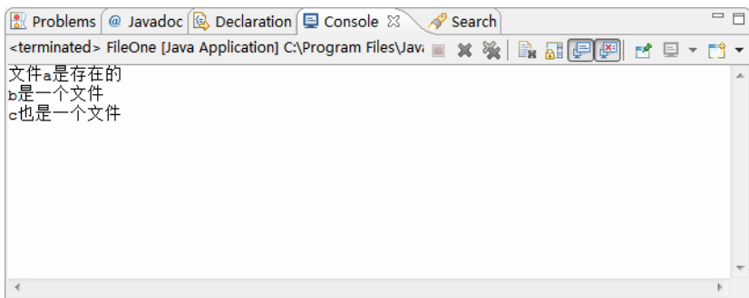
图 11-16 文件类
