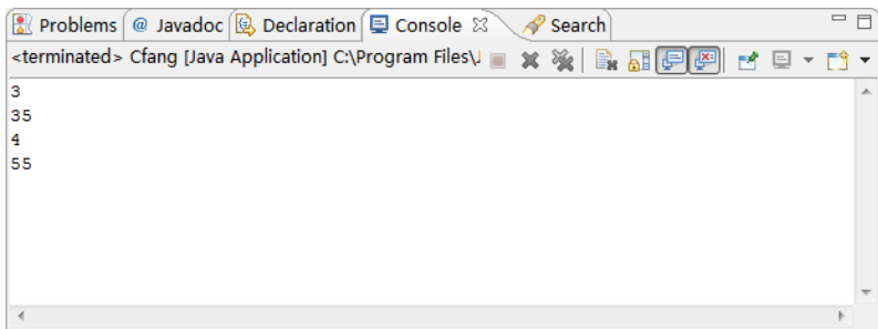
图 9-13 重载的规则
