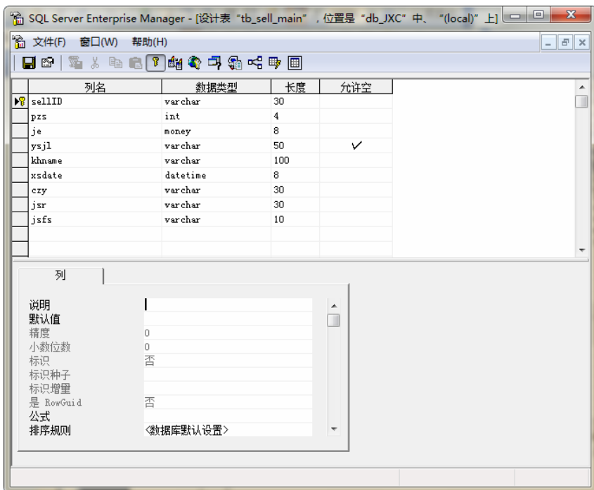
图 19-10 销售主表
