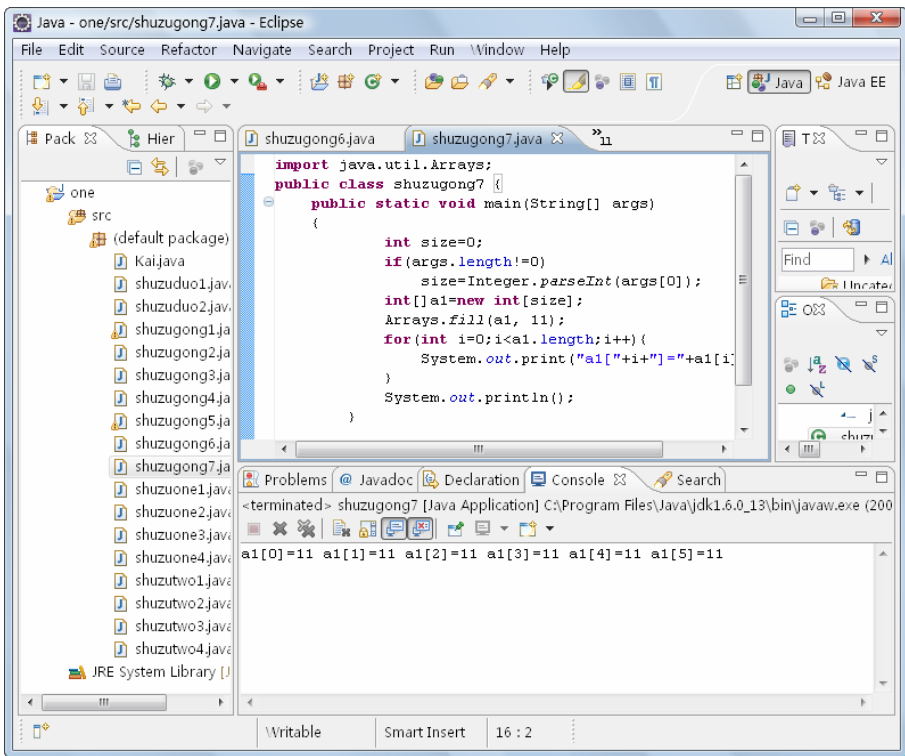
图 7-22 运行结果
