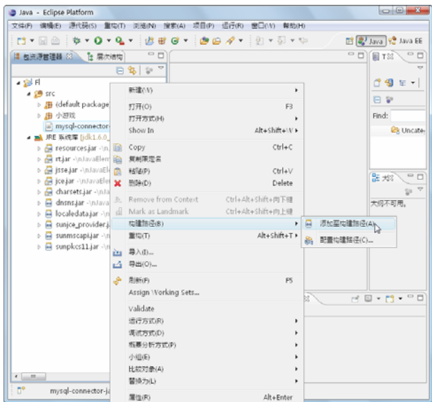
图 17-7 选择命令
