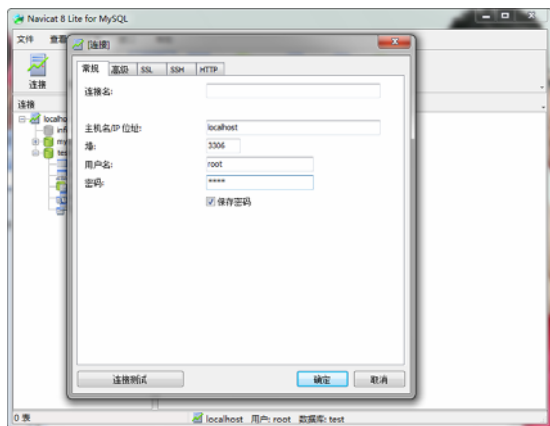
图 16-1 “连接”对话框
