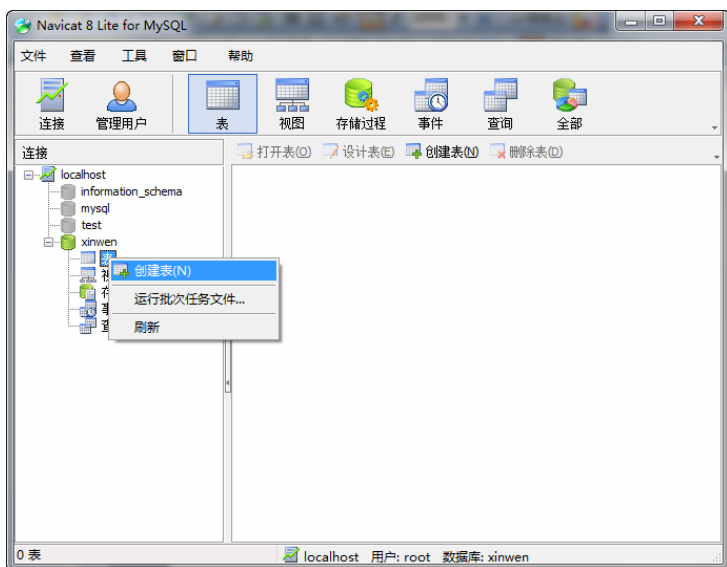
图 16-25 选择命令
