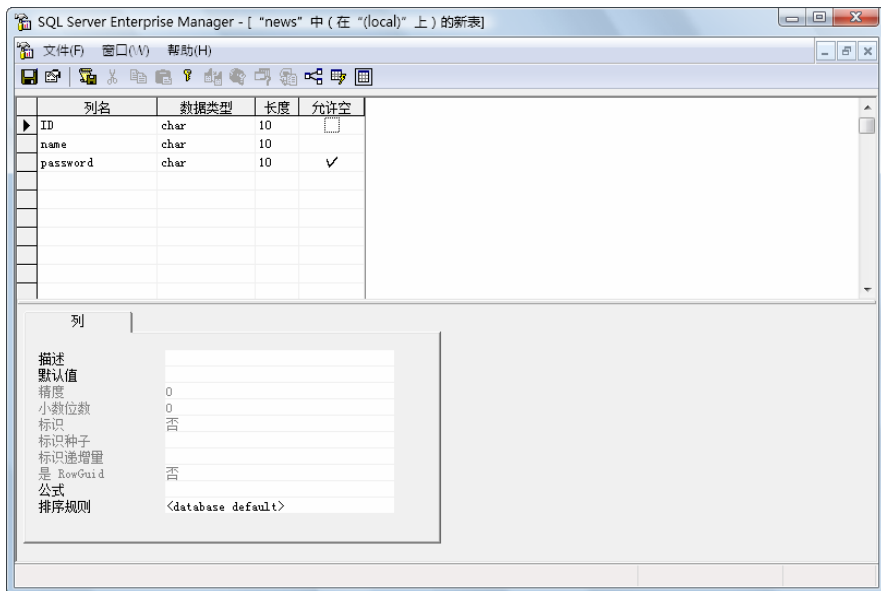
图 16-36 设置字段
