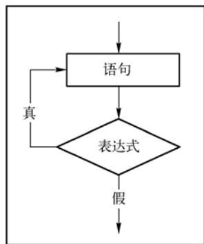
图 6-14 do...while 流程图
