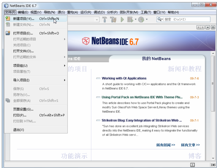
图 2-28 新建项目
