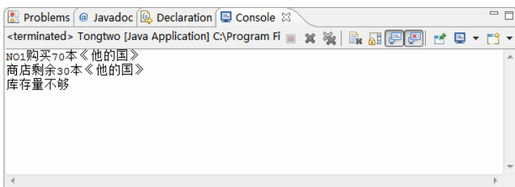
图 12-16 实现同步
