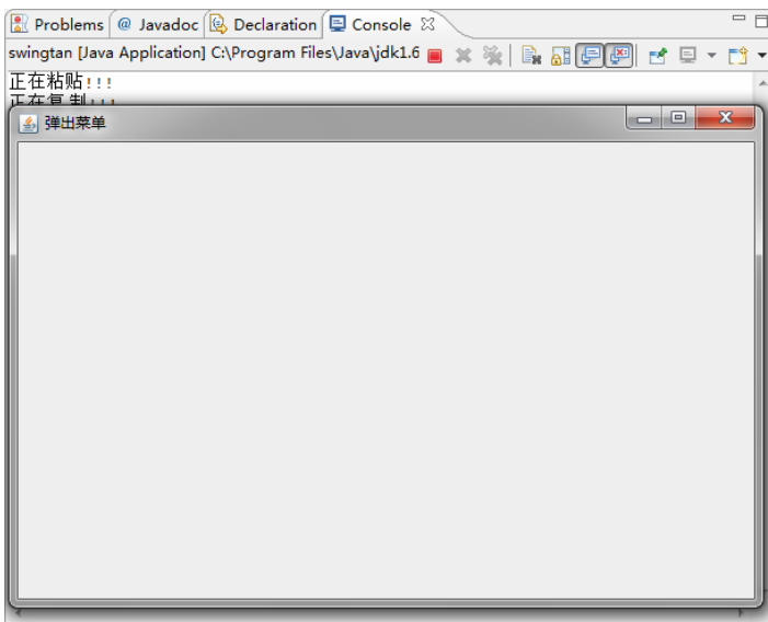
图 15-5 执行结果
