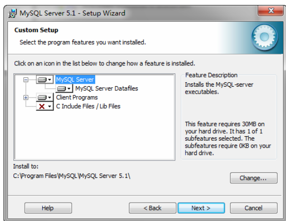
图 16-10 安装位置
