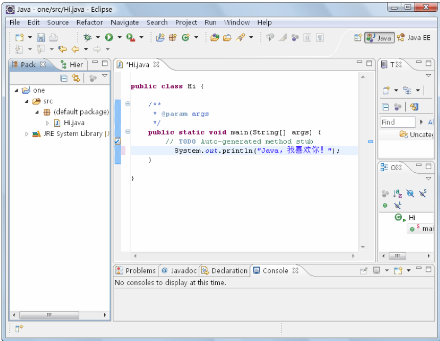
图 2-13 输入代码
