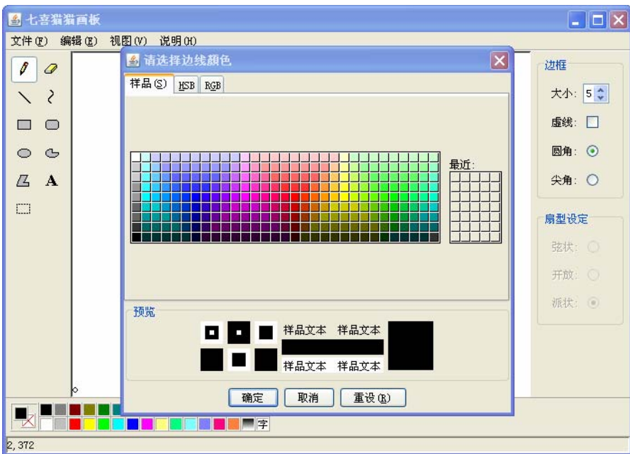
图 18-8 自定义颜色
