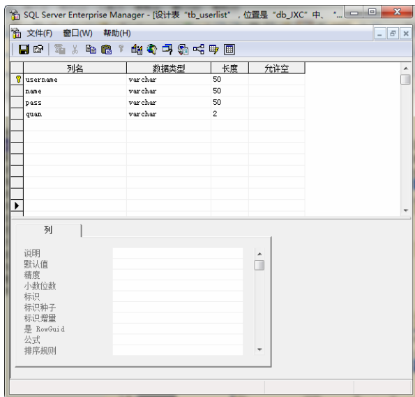
图 19-5 表 tb-userlist
