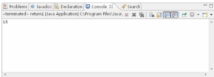
图 6-25 程序结果
