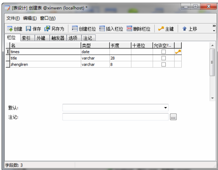
图 16-26 创建字段
