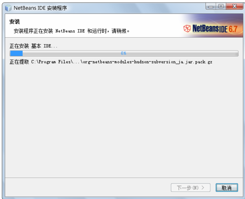
图 2-25 安装 Netbeans
