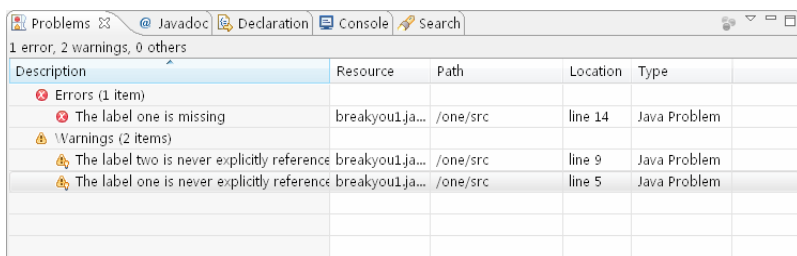
图 6-24 提示的错误
