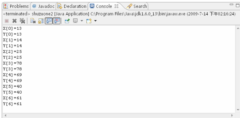
图 7-3 一维数组
