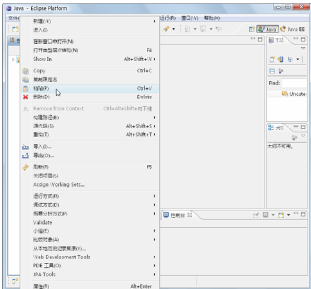
图 17-6 复制与粘贴
