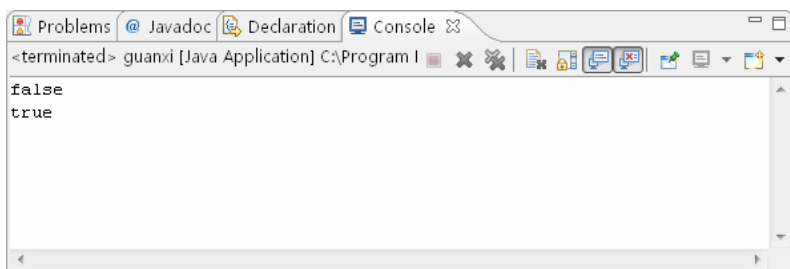
图 4-9 关系运算符
