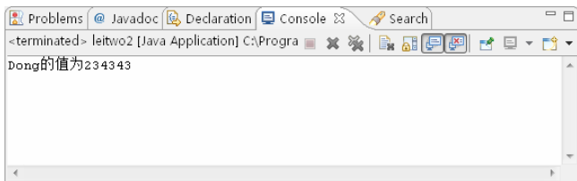
图 8-6 public 修饰符
