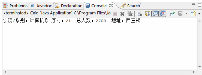
图 9-8 重写
