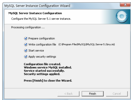
图 16-21 安装完成
