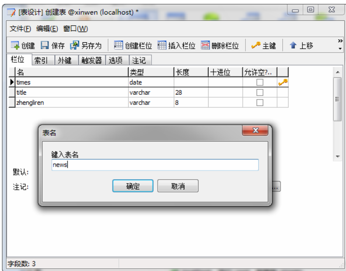
图 16-27 输入表名
