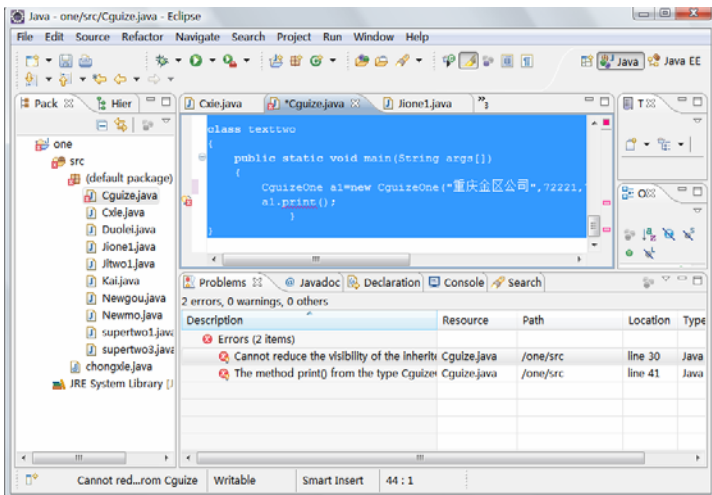
图 9-9 重写的规则
