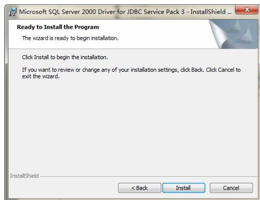
图 19-20 安装
