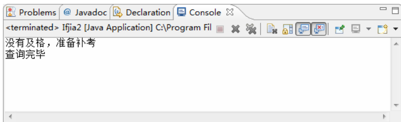
图 5-6 条件语句
