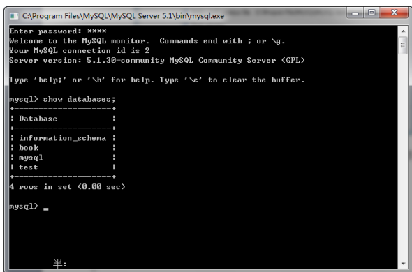
图 16-22 管理工具
