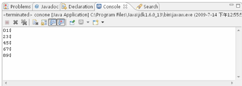
图 6-27 运行结果
