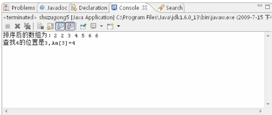
图 7-17 搜索数组
