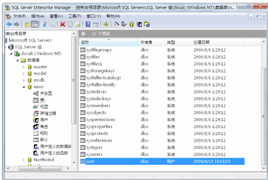
图 16-38 新建表
