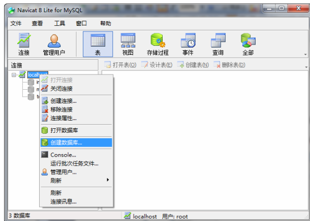
图 16-23 选择命令
