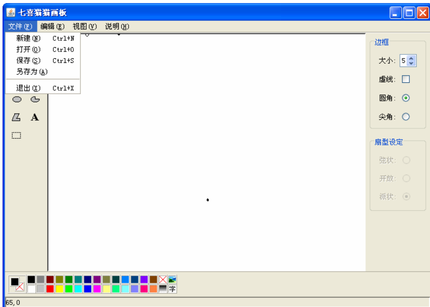
图 18-3 菜单命令
