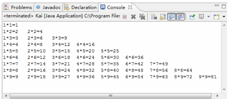
图 6-8 九九乘法表
