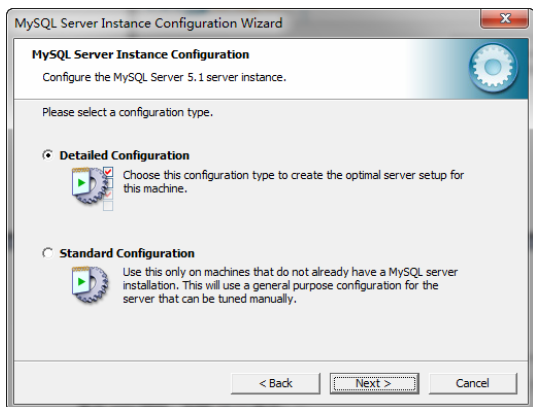
图 16-15 完全设置
