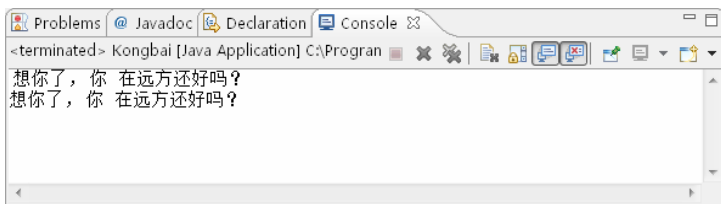
图 4-26 去除空白
