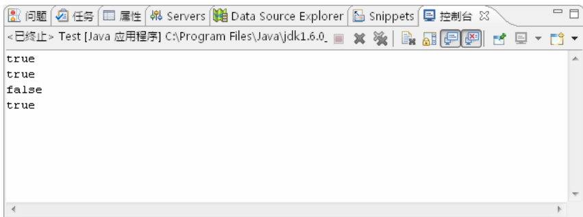
图 3-1 常量
