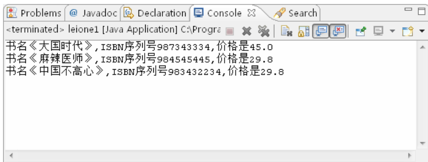
图 8-3 构造方法
