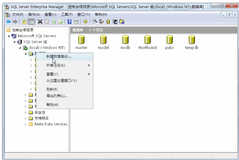
图 16-31 新建数据库
