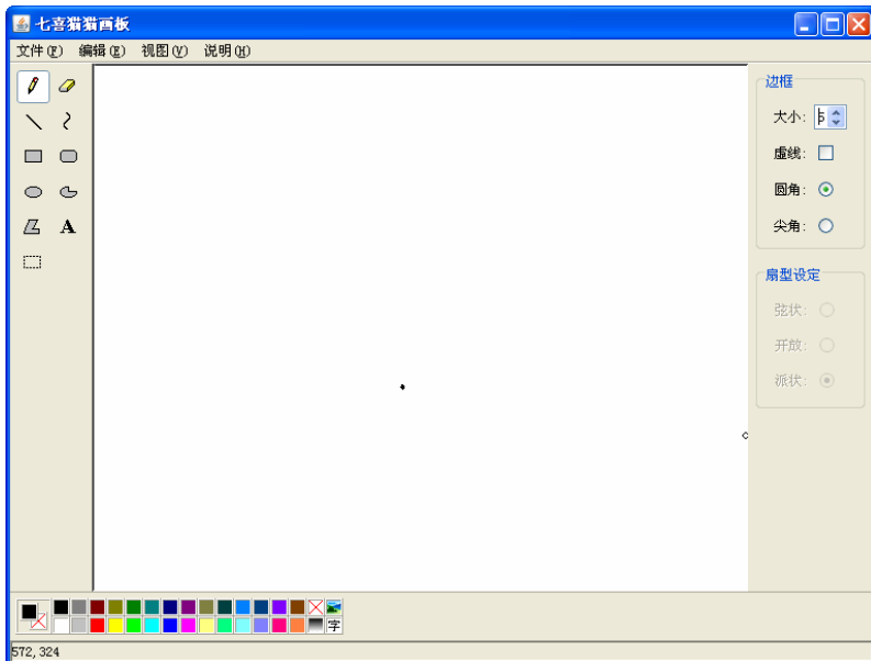
图 18-1 软件界面
