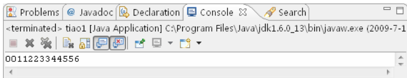
图 6-29 执行结果
