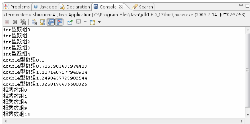
图 7-6 初始化数组
