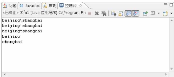
图 3-7 运行的结果
