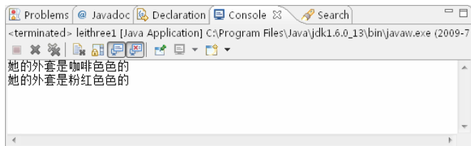
图 8-11 this 的使用
