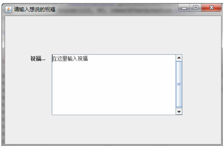
图 15-13 执行结果
