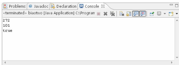
图 4-15 表达式
