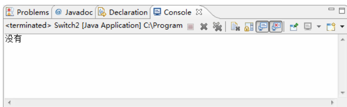
图 5-12 执行结果
