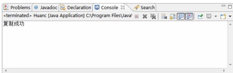
图 11-11 复制成功
