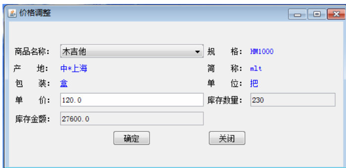
图 19-34 价格调整
