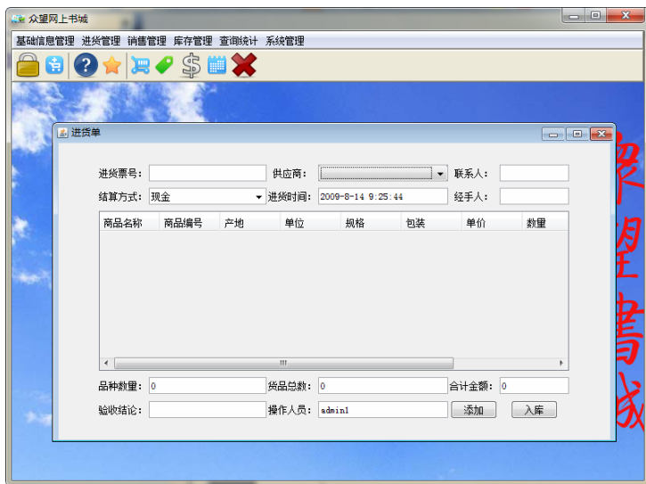
图 19-4 操作数据库
